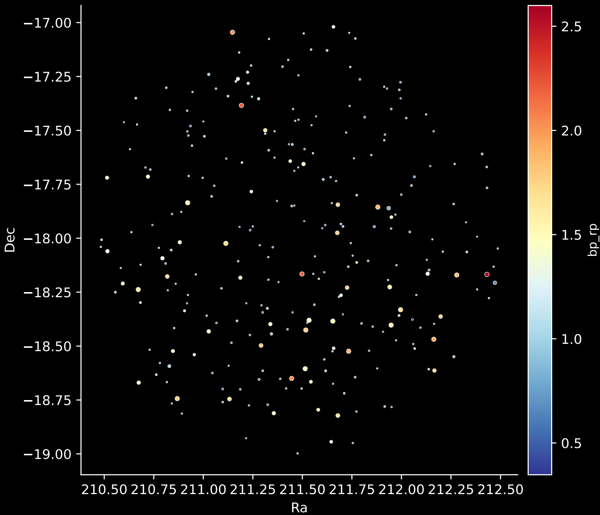
GALAH DR4 Field: [8618] Stars: 271
