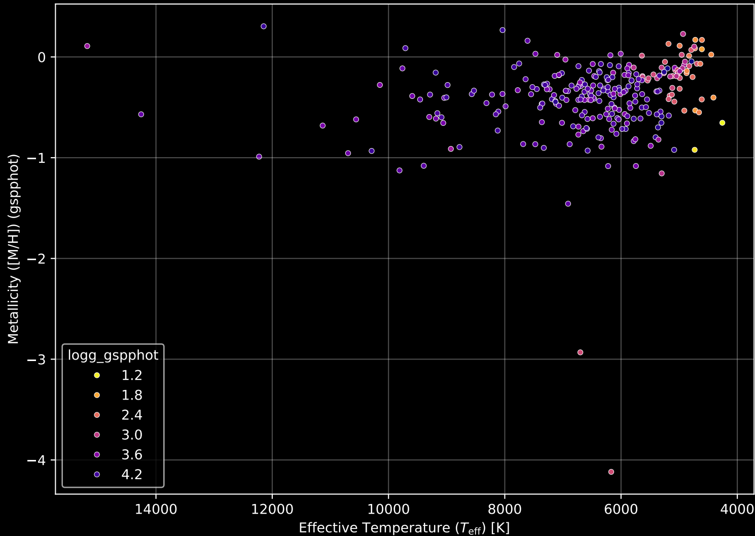
GALAH DR4 Field: [8618] Stellar Population Parameters (n= 271)
