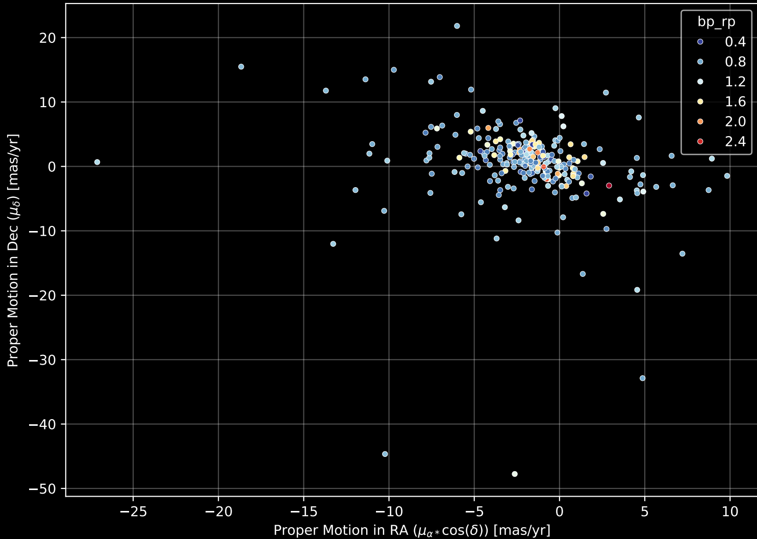
GALAH DR4 Field: [8618] Proper Motion Diagram (n= 271)
