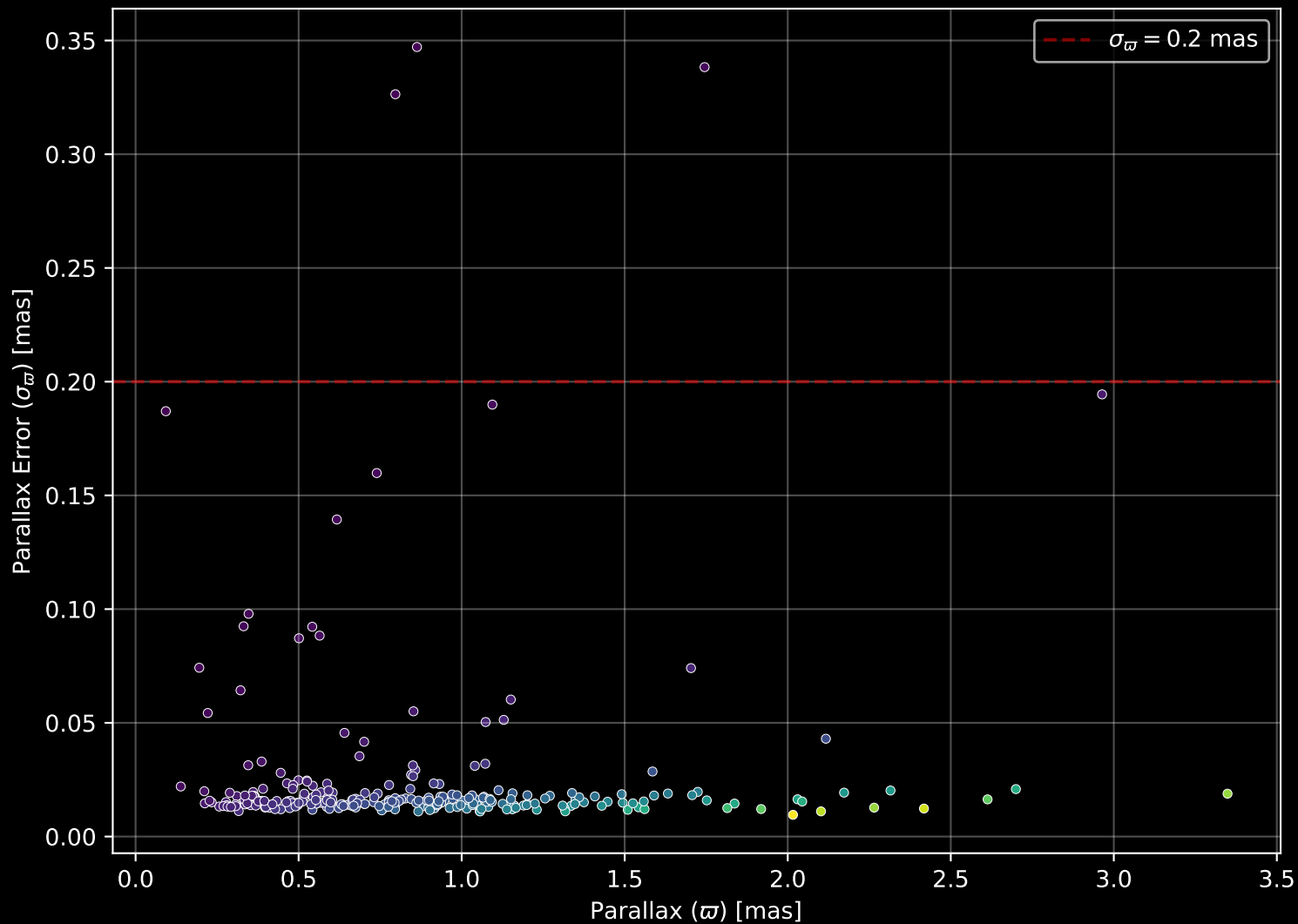
GALAH DR4 Field: [8618] Parallax Quality (n= 271)
